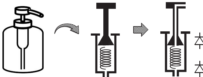
図6 シャンプーポンプの構造の考え方
